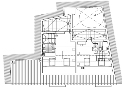
PLANTA BAJO CUBIERTA
