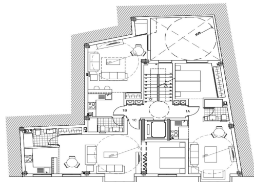
PLANTA PRIMERA
